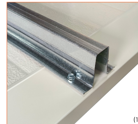
(1) Omega de reforço galvanizado (1) Omega de refuerzo galvanizado
