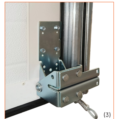
(3) Paraquedas de cabo galvanizado (3) Paracaídas de cable galvanizado
