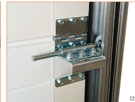
(2) Dobradiça lateral e porta-rodízio galvanizados (2) Bisagra lateral y porta rodillo galvanizado
