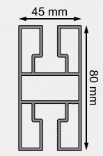
Pilar Intermédio Pilar Intermedio
