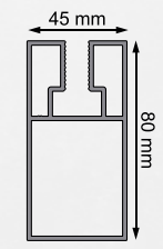
Pilar Exterior Pilar Externo
